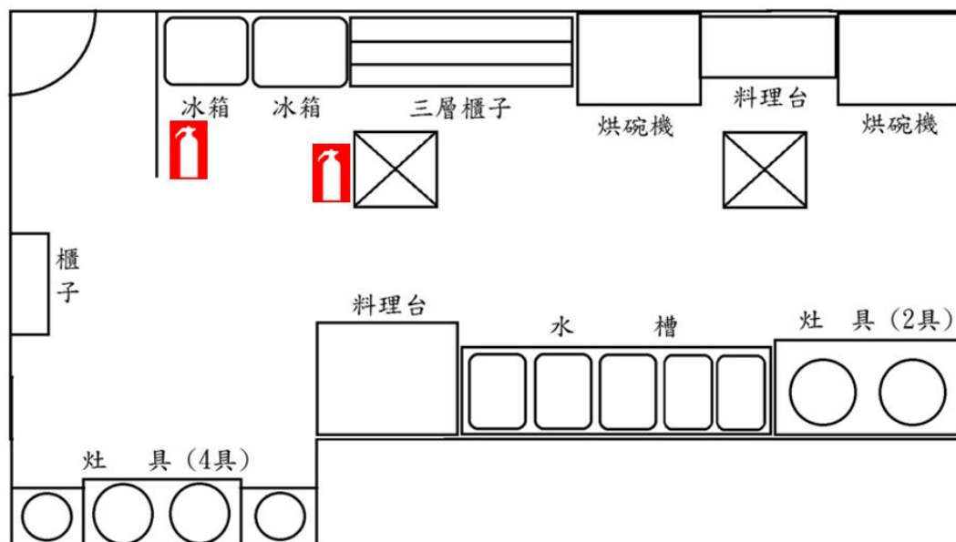
平面圖
